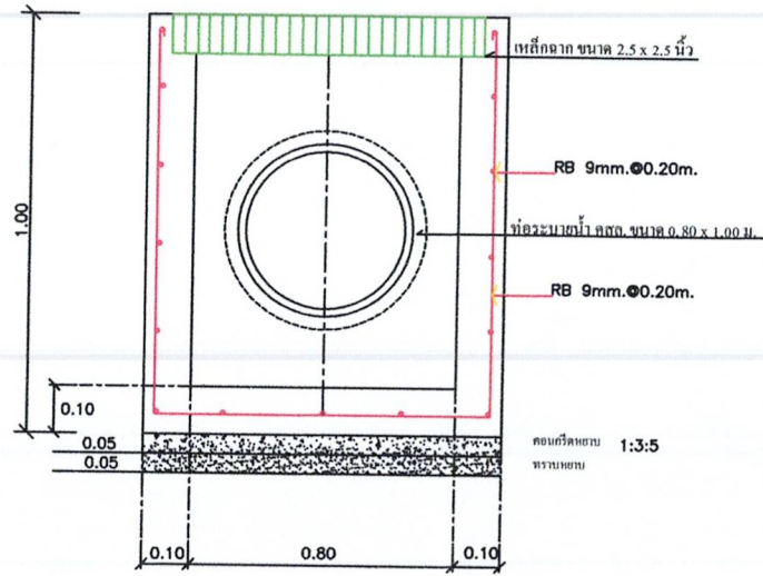
รูปตัดขยายบ่อพัก 2 SCALE not
