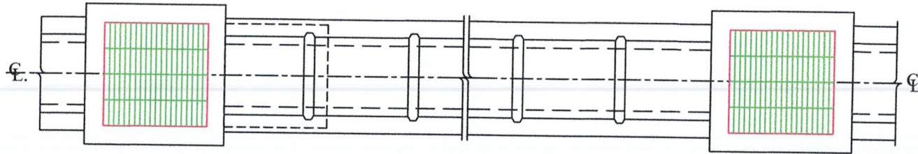
แปลนแนวท่อและบ่อพักน้ำ
