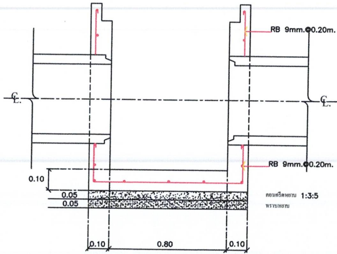
รูปตัดขยายบ่อพัก 1 SCALE not
