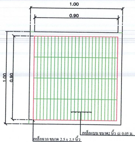
แปลนฝาบ่อพัก SCALE not
