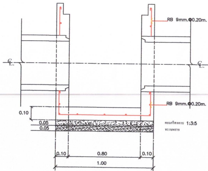
รูปตัดขยายบ่อพัก 1 SCALE not
