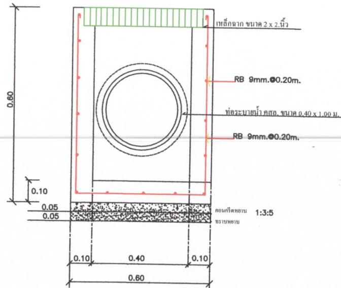
รูปตัดขยายบ่อพัก 2 SCALE not
