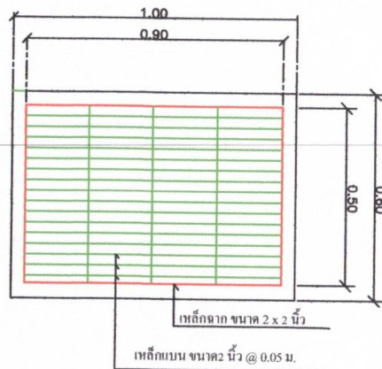
แปลนฝ้าบ่อพัก SCALE not
